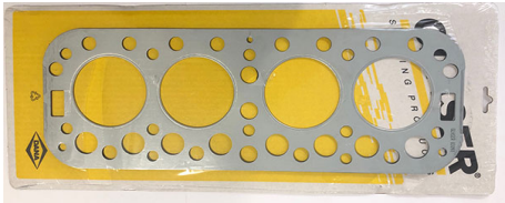
Joint de culasse Peugeot 403 Réf 170575 en rupture
