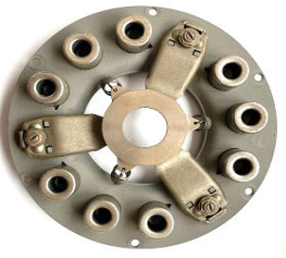
Mécanisme embrayage PEUGEOT 403 DIESEL Réf 30026
