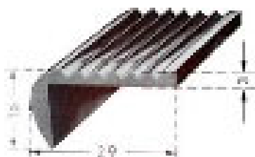
Cornière bombée striée Longueur 1m66 Réf 140341
