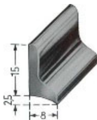
Profil de marchepied Longueur 1m66 Réf 140345
